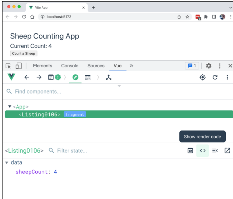
FIGURE 1-4: The Vue DevTools extension.
